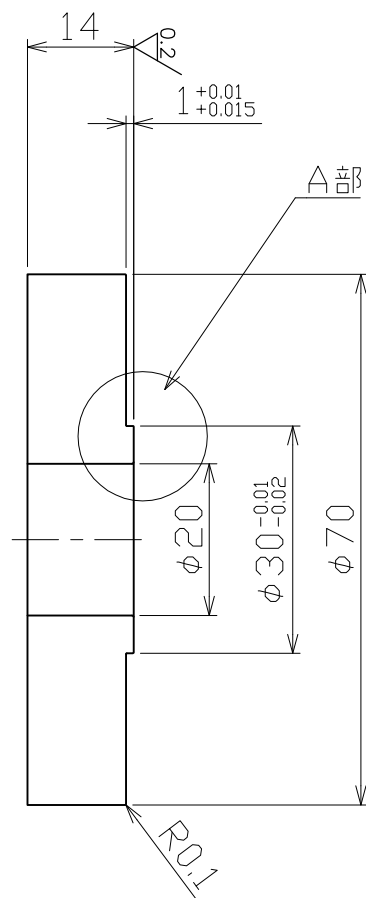
① 部品詳細図
