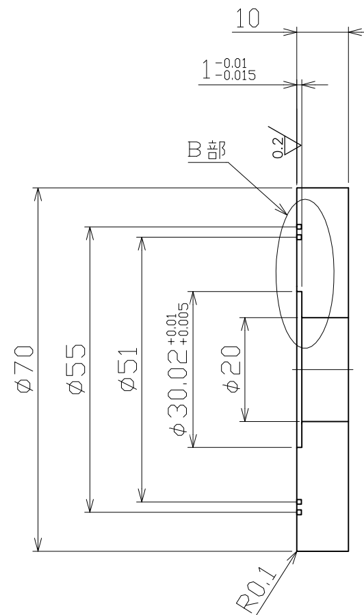
② 部品詳細図
