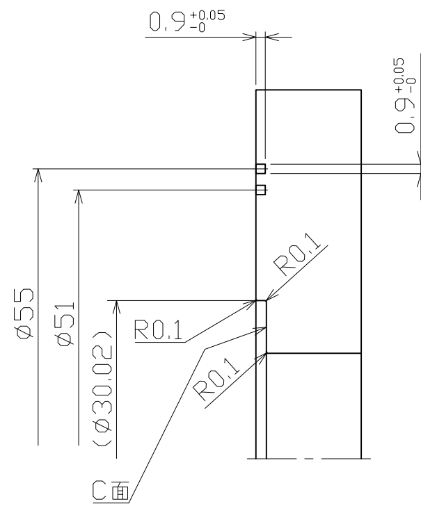
B部詳細図
