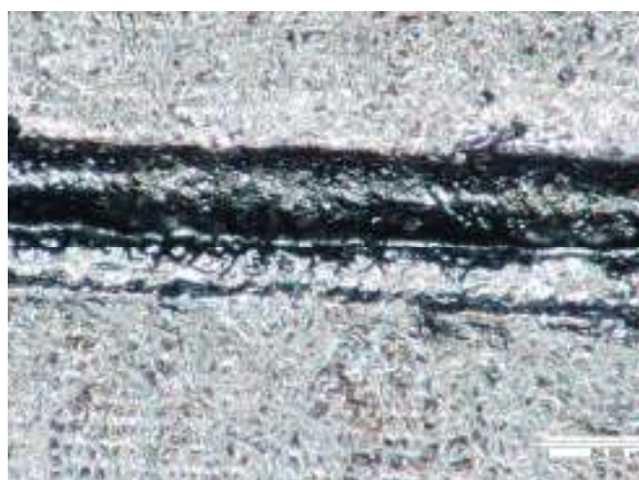
No.4-ab外面
