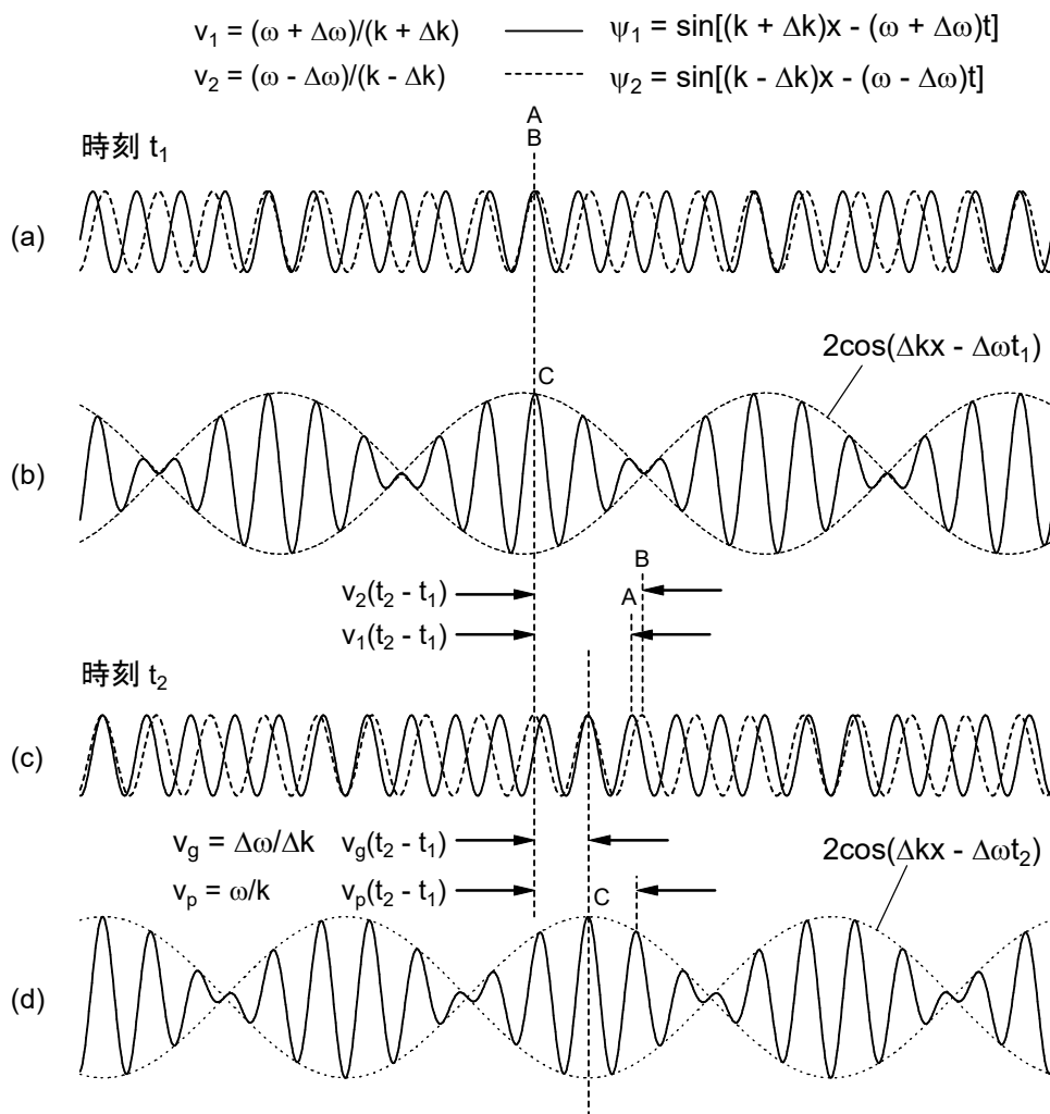
図1. (a) 時刻 t_1 での2つの carrier wave. (b) 時刻 t_1 での modulation envelope. (c) 時刻 t_2 での2つの carrier wave. A, B は(a)での A, B からの移動位置を表す。(d) 時刻 t_2 での modulation envelope. C は(b)での C からの移動位置を表す。 (E. Hecht, Optics , 3rd ed., Addison Wesley, Reading, 1998, p.298, Fig. 7.15を参考に作成。)
