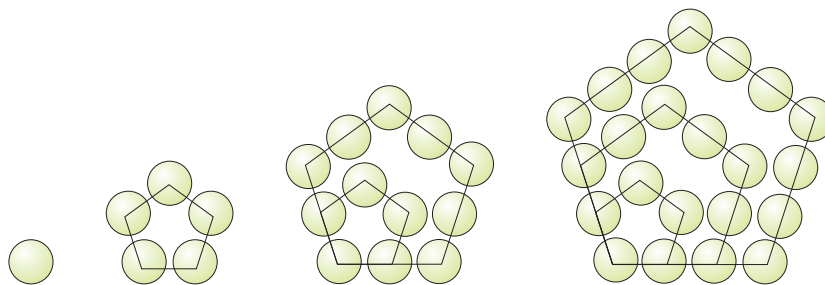
図3 五角数
