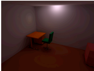
(g) 提案手法による照度分布
