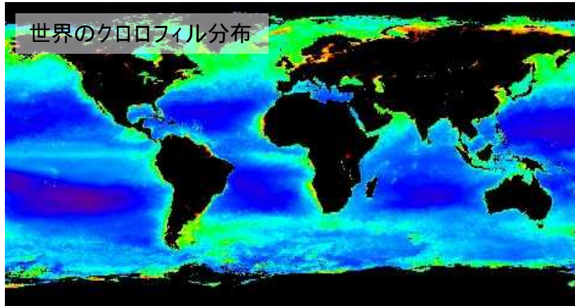
出典 : NASA, http://oceancolor.gsfc.nasa.gov/PRODUCTS/
